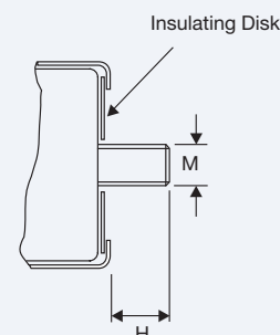
ALS31 Stud Mounting
