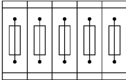
Sicherungsklemmen in Verbundanordnung, Block bestehend aus 5 Sicherungsklemmen
