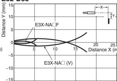
E32-D33
