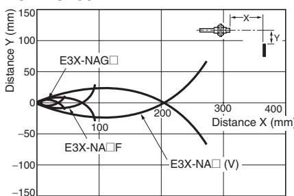
E32-DC200
