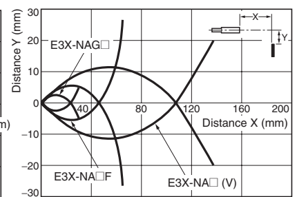
E32-D11R/D12R
