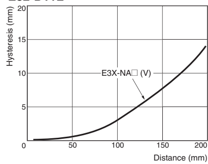
E32-D11L
