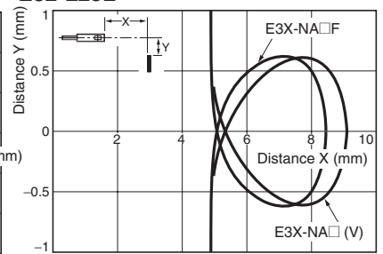
E32-L25L
