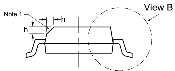
View A-A
