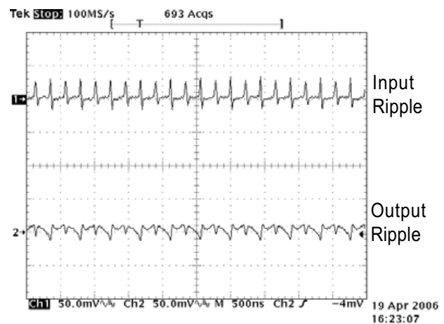
Ripple 2X Flash 1000mA, V_{IN}=3.6V
