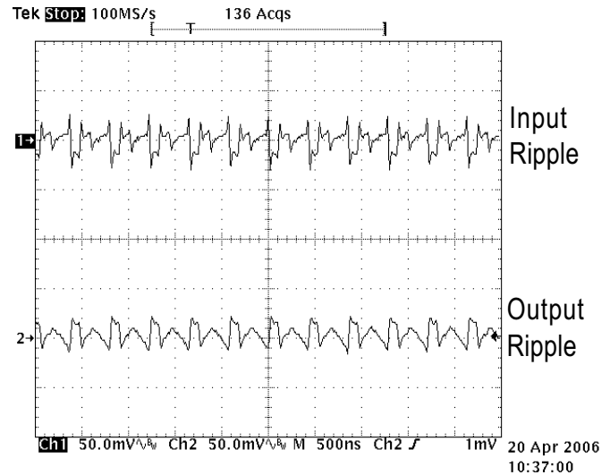
Ripple 2X Flash 700mA, V_{IN}=3.6V
