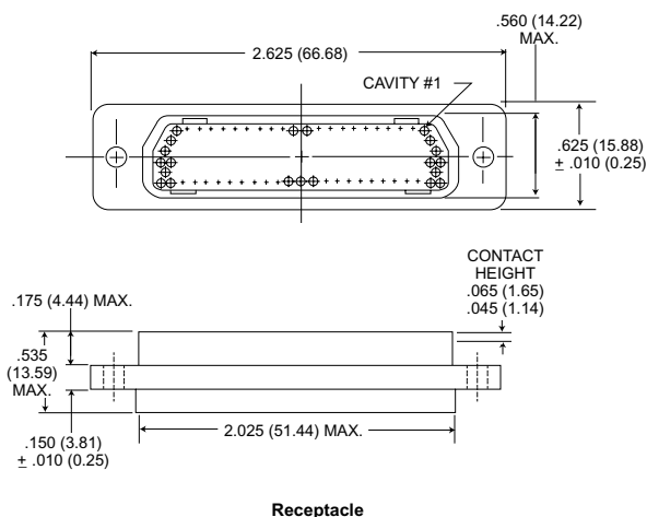
Receptacle
