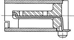
A-A (10:1) (CONTACT No. 1, 10)
