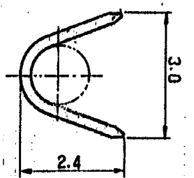
断面 B-B
