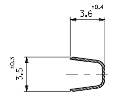
断面 B-B SECT.B-B
