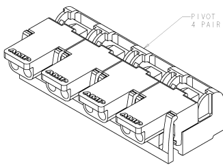
1339376-2 SHOWN SCALE 4:1
