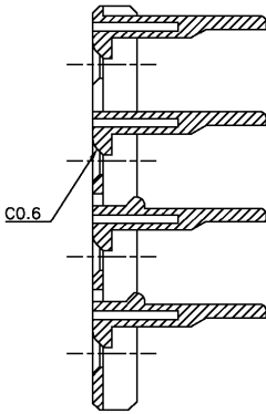
SECT A-A
