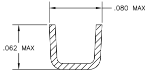
SECTION A-A SCALE 20:1
