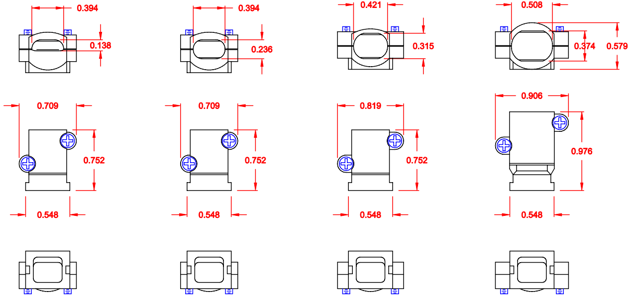
P/N 955-09-SR-4-7 CABLE RANGE = 0.157 - 0.276
