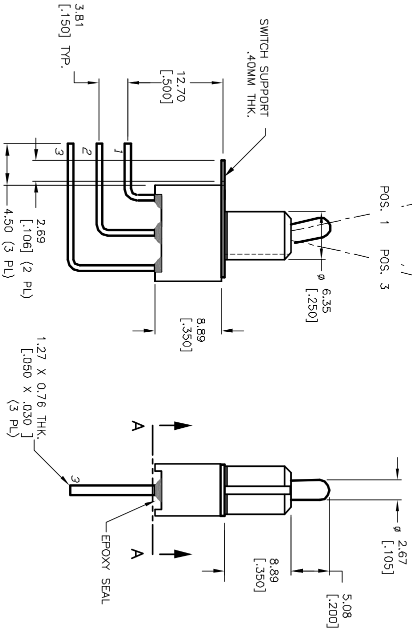
SECTION A-A
