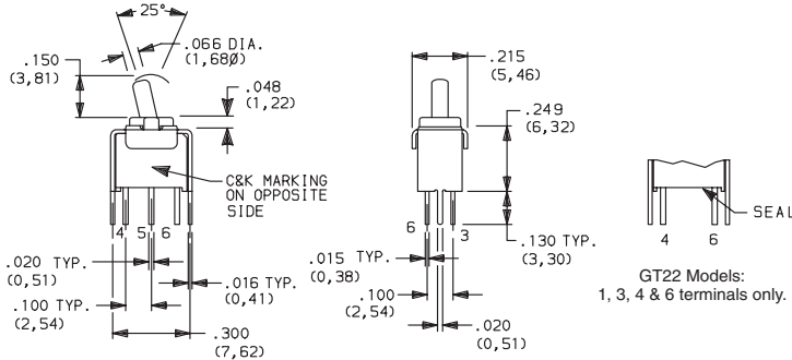
GT21MV3XE DPDT
