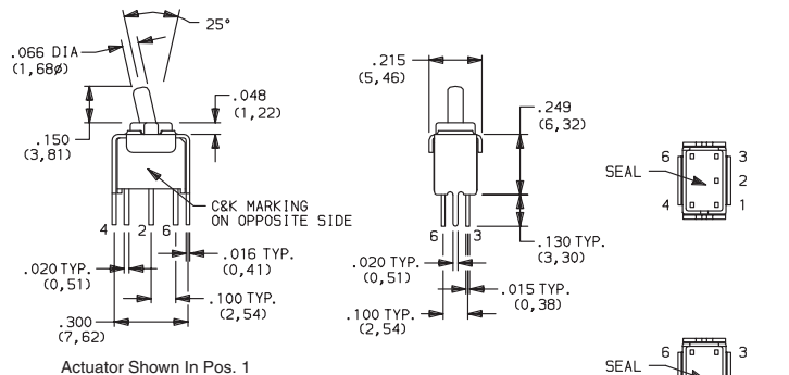
Actuator Shown In Pos. 1
