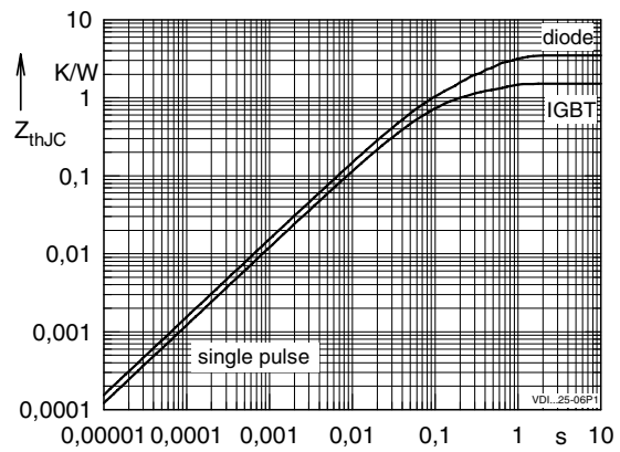
Fig. 12 Typ. transient thermal impedance RBSOA
