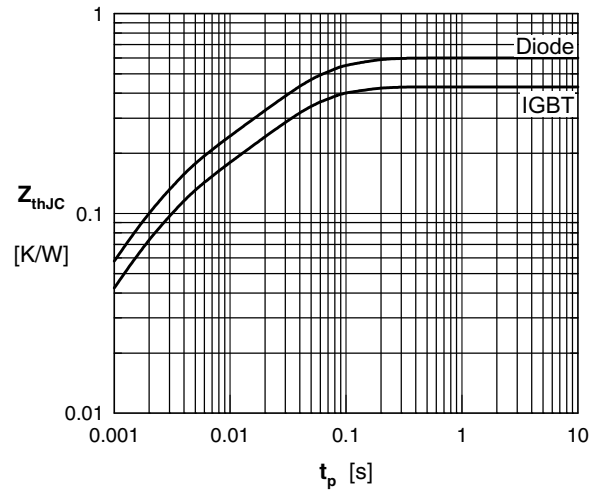
Fig. 14 Typ. transient thermal impedance
