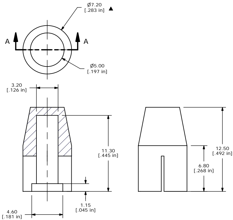
SECTION A-A SCALE 4 : 1
