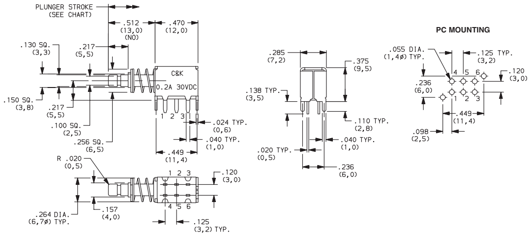
PN21LASA03QE DPDT
