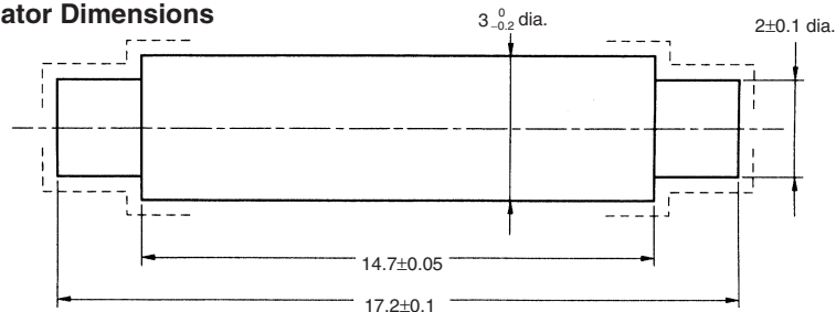
Actuator Dimensions
