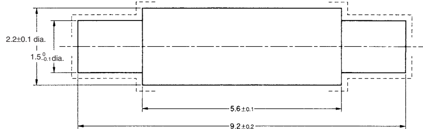
Actuator Dimensions
