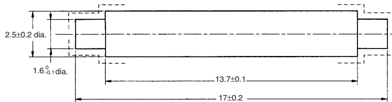
Actuator Dimensions
