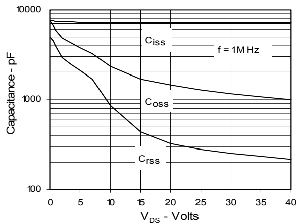
Fig. 11. Capacitance
