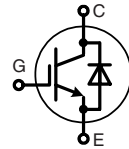
IXEN 60N120D1
