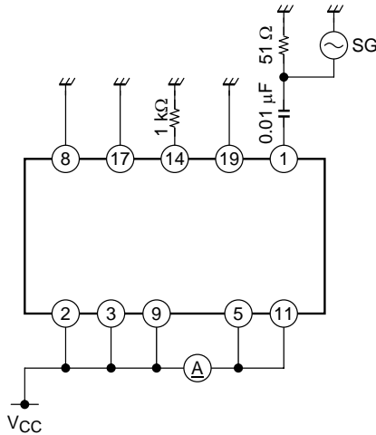
I_{ccqfm}
