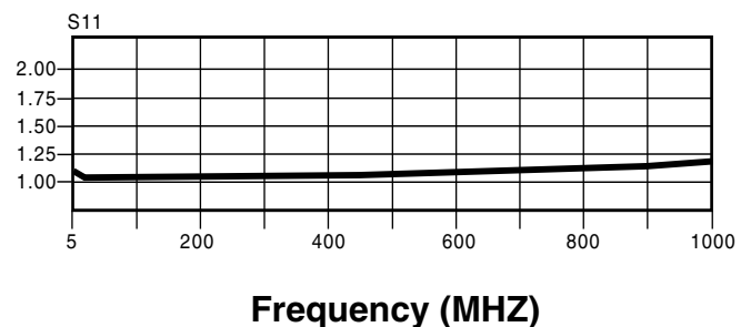
INPUT VSWR
