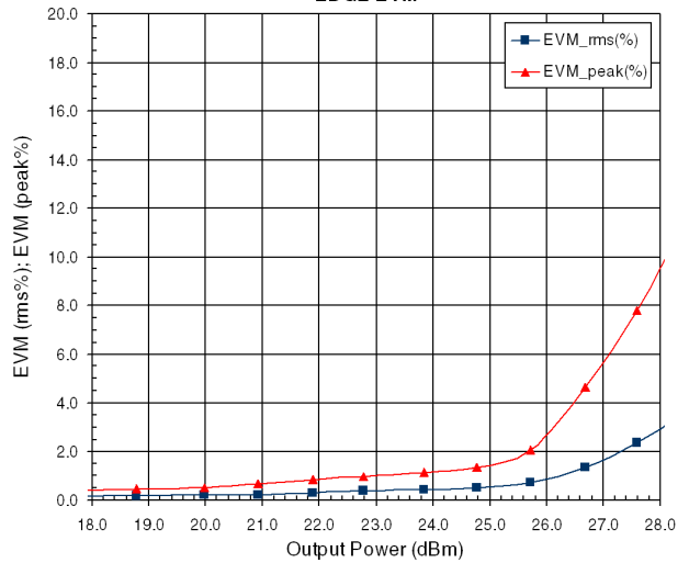
RF3807412 @ 940 MHz EDGE EVM
