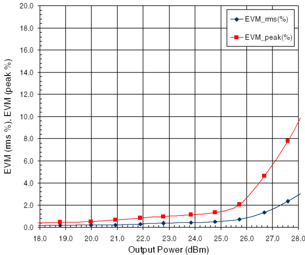
RF3807412 @ 940 MHz EDGE EVM
