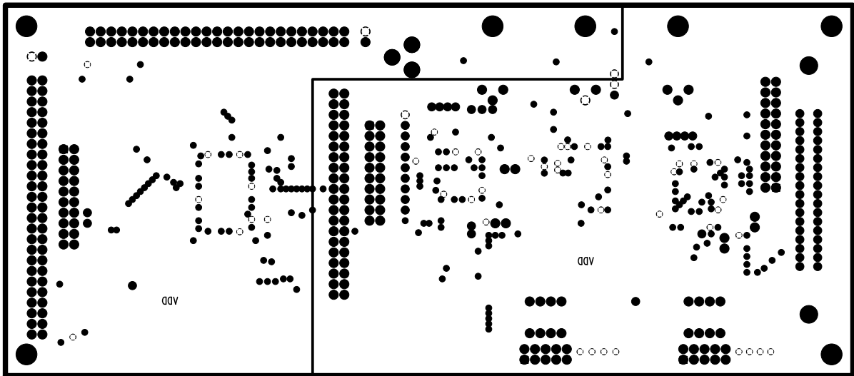
POWER PLANE LAYER 4 (DB654CE.pho)
