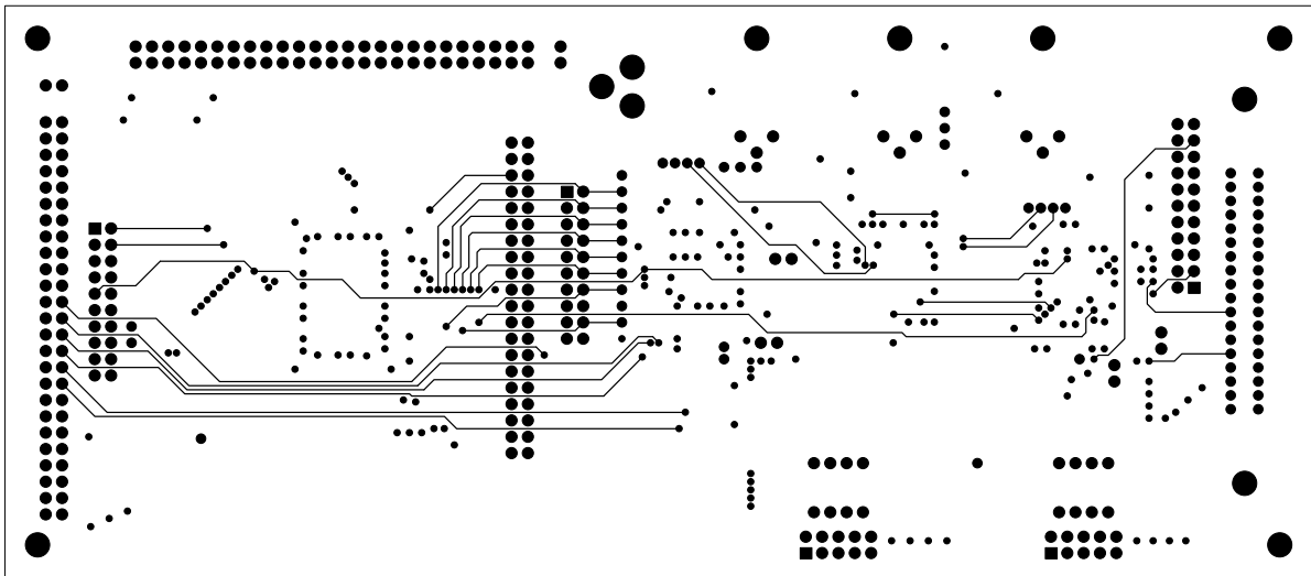
SIGNAL LAYER 3 (BB854CE.pho)
