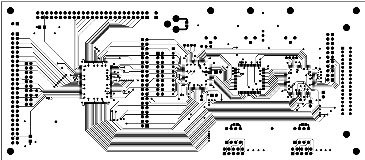
TOP Layer 1 (AB6624CE.pho)
