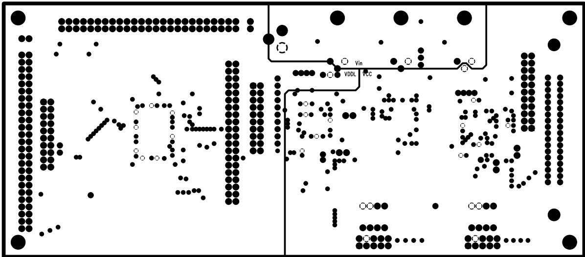
POWER PLANE LAYER 5 (EB6624CE.pho)
