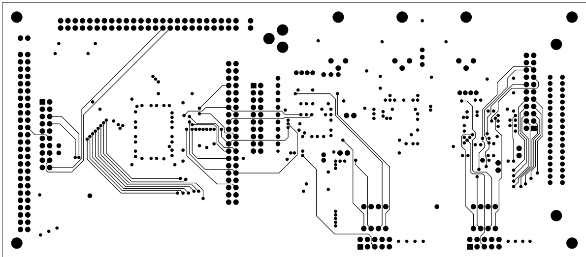
SIGNAL LAYER 7 (GB6624CE.pho)
