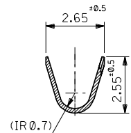
断面 A-A SECT.A-A
