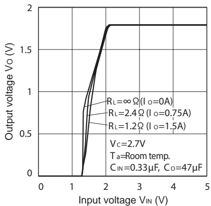
Fig.15 Output Voltage vs. Input Voltage (PQ018EZ1HZxH)
