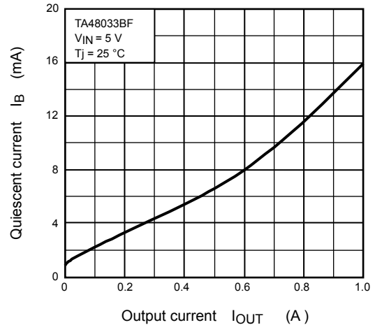
I B - I OUT
