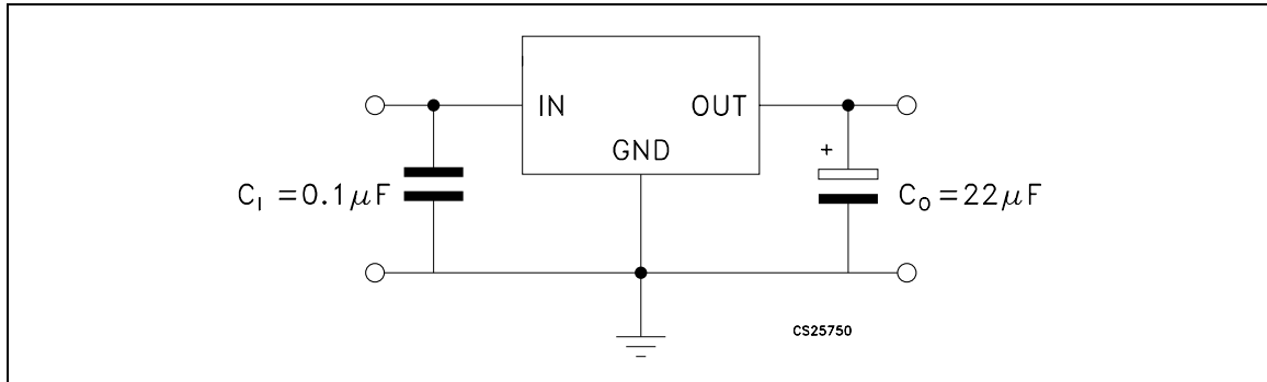
Figure 3. DC Parameters
