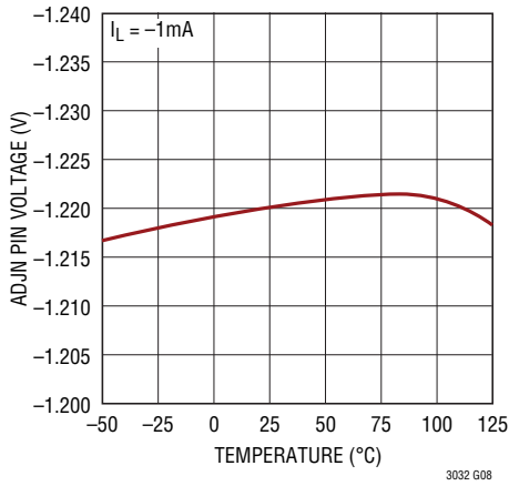
LT3032 ADJN Pin Voltage
