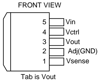
TO263-5L
