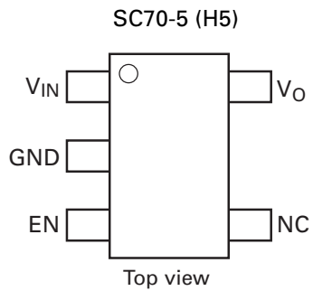
ZXCLxxx
