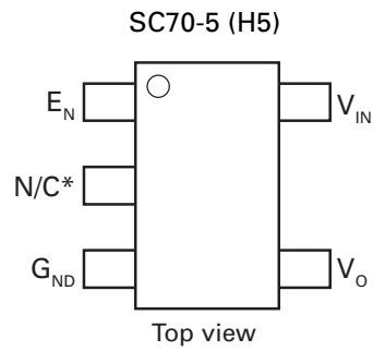
ZXCL5213Vxx
