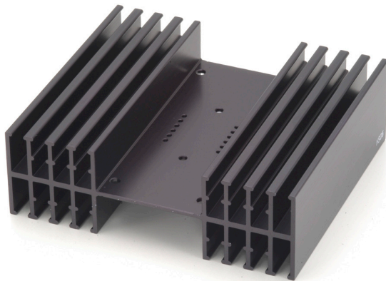
HS06 0.96°C/W
