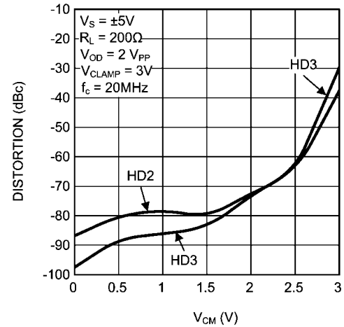
Distortion vs. V_{CM} ( f_c=20MHz , R_L=200\Omega )
