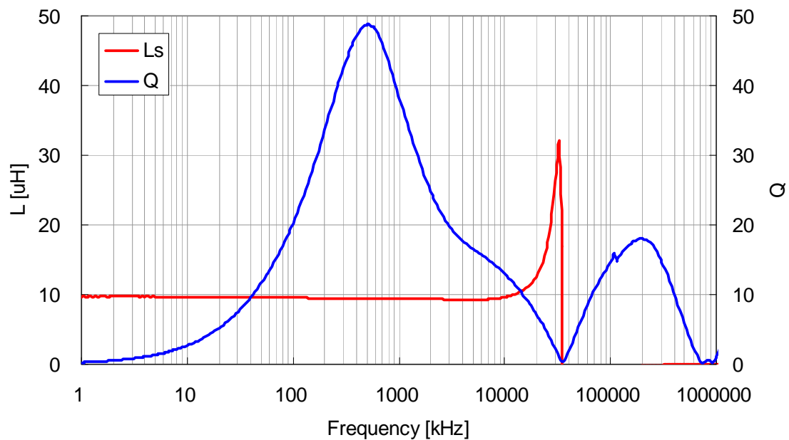
VLF4014ST-100M1R0
