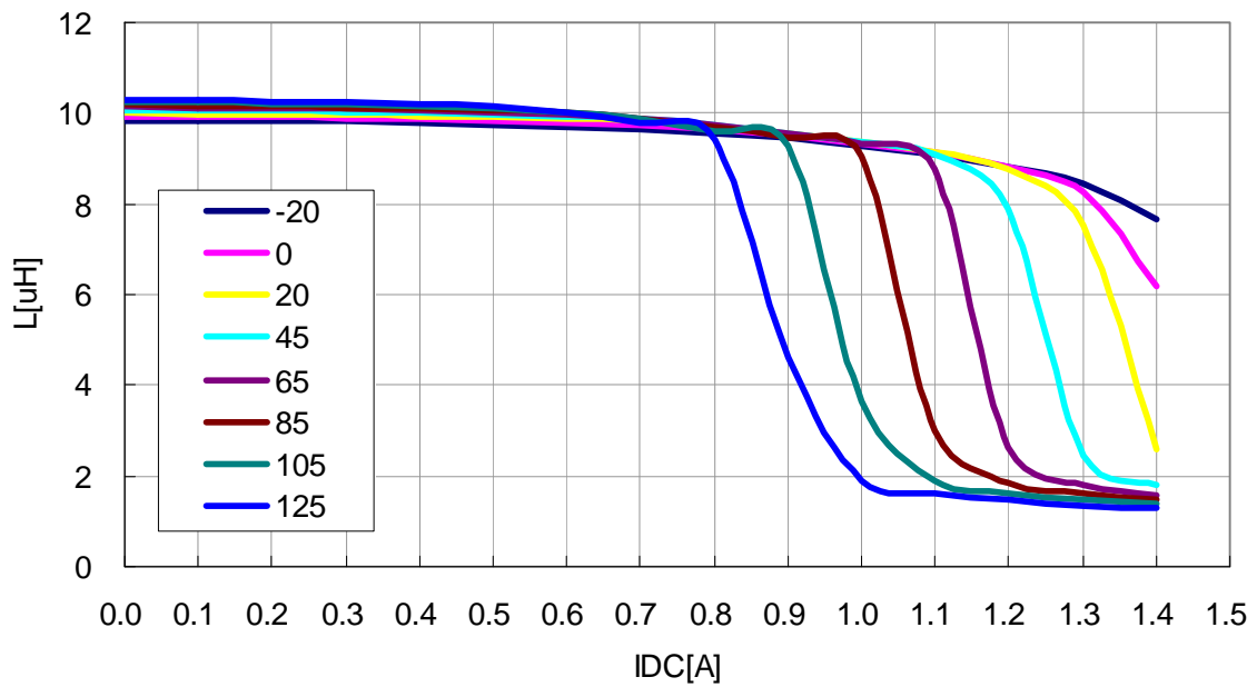
VLF4014ST-100M1R0
