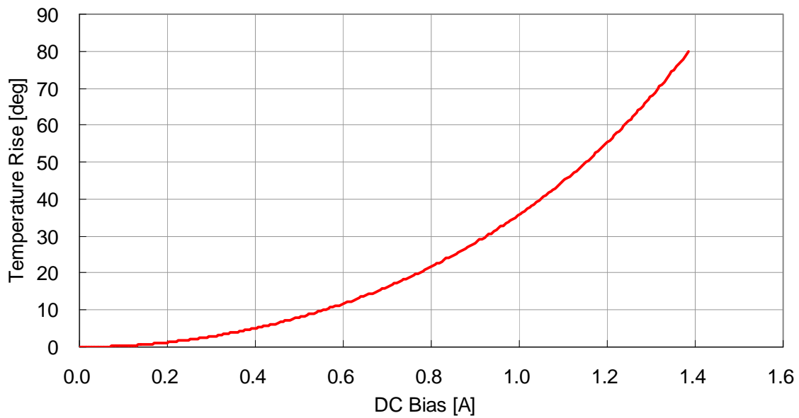
VLF4014ST-100M1R0
