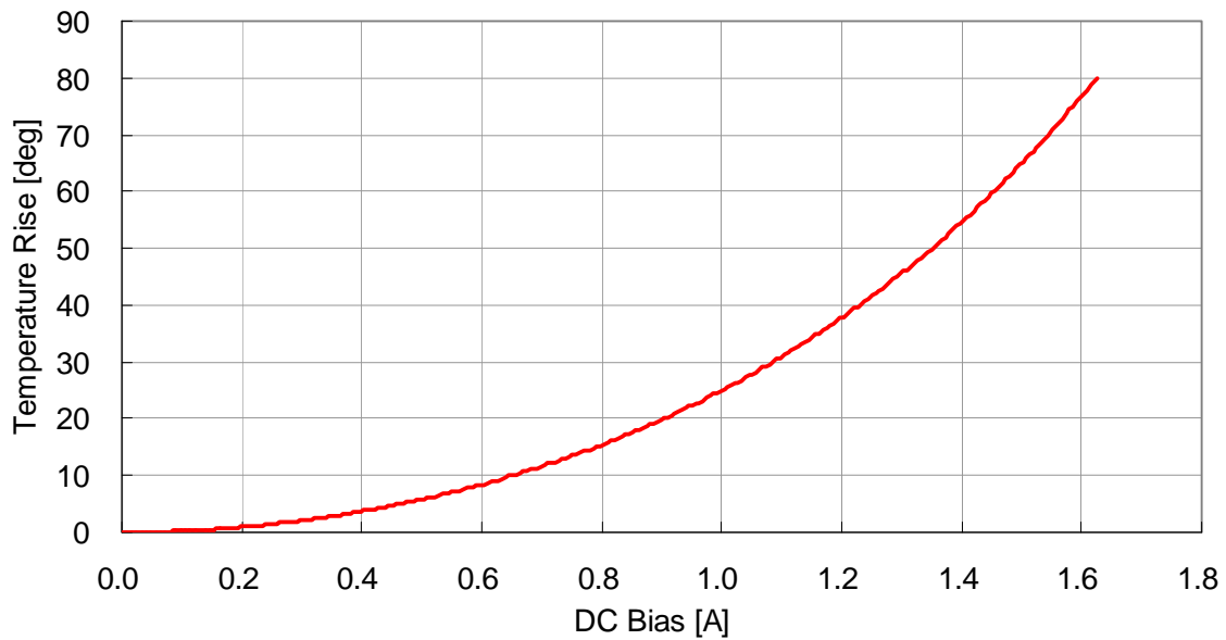
VLF4014ST-100M1R0
