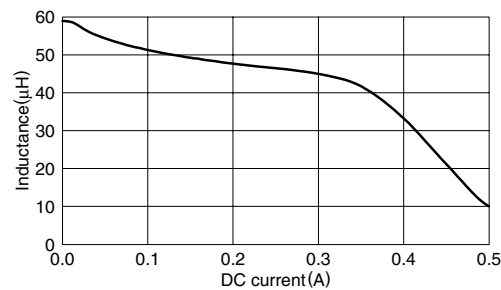
VLF4012AT-470MR30
