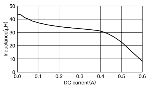
VLF4012AT-330MR39
