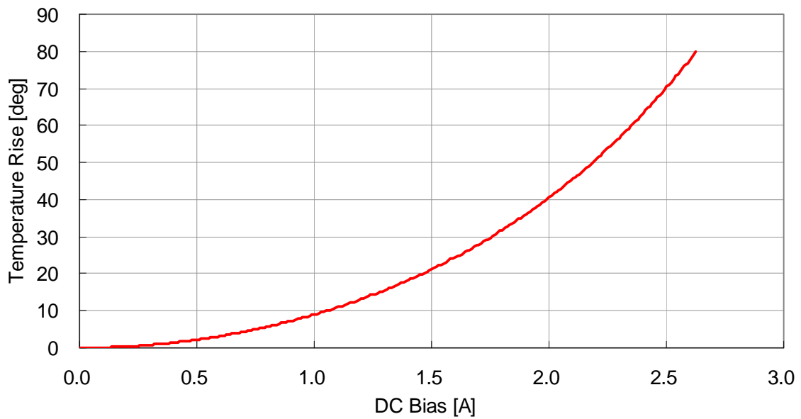
VLS3012T-1R5N1R7
