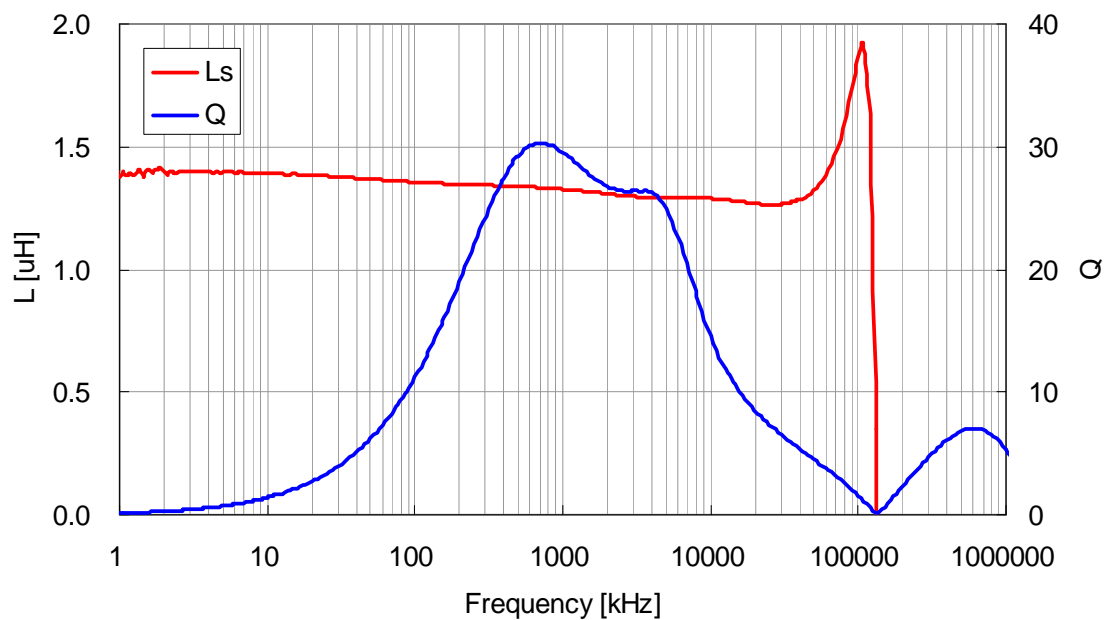
VLS3012T-1R5N1R7
