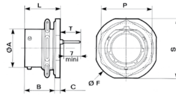
Version à picots droits PC tail version
