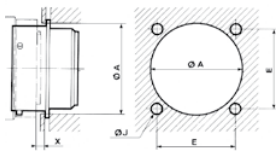
Embase à collerette carrée Square flange receptacle
