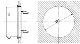
Embase à collerette ronde Solder fixing receptacle
