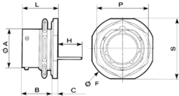
Version pour connexions enroulées (WW) Wire-wrap version
