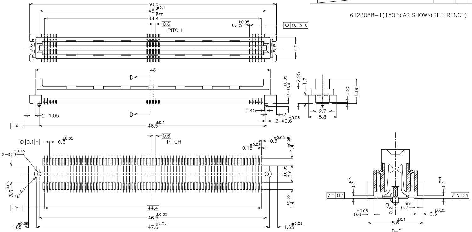
参考基板取り付け寸法 REFERENCE P.C.BOARD LAYOUT
