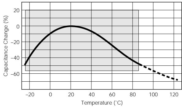
Char. SL/GP
