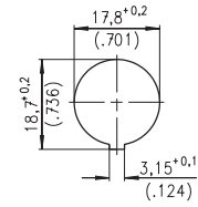
Montageausschnitt
