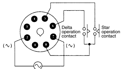
H3CR-G8L
