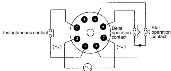
H3CR-G8EL
