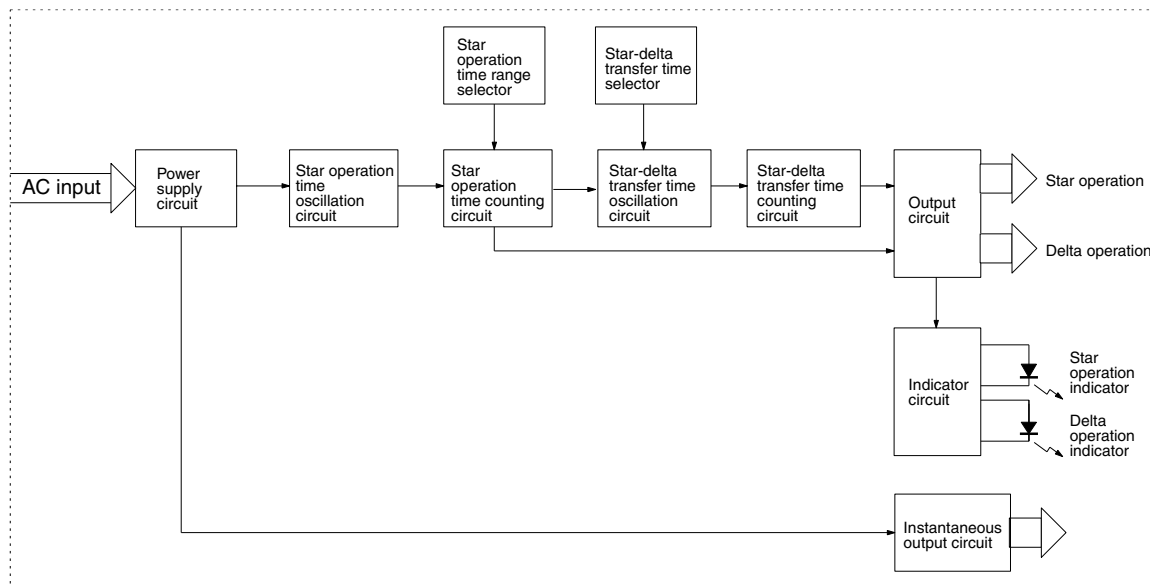
H3CR-G8EL
