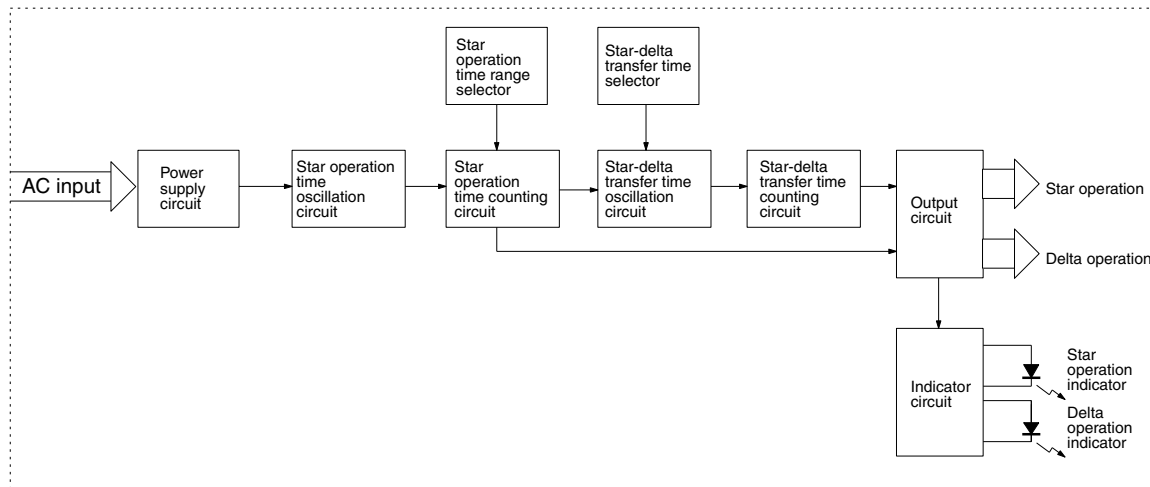
H3CR-G8EL
