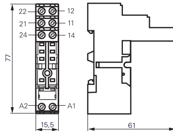
S0416-AB
