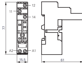
S0416-AA
