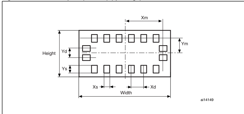
Figure 7. MEMS footprint (LGA16 (D) package)
