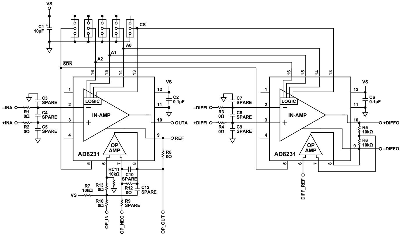
Figure 3. AD8231-EVALZ Schematic
