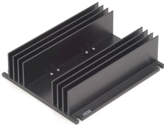
HS18 1°C/W
