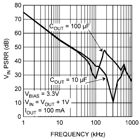
V_{IN} PSRR
